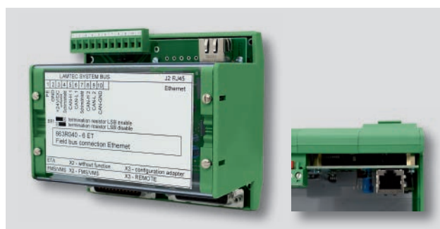
Bus de terrain Ethernet.
