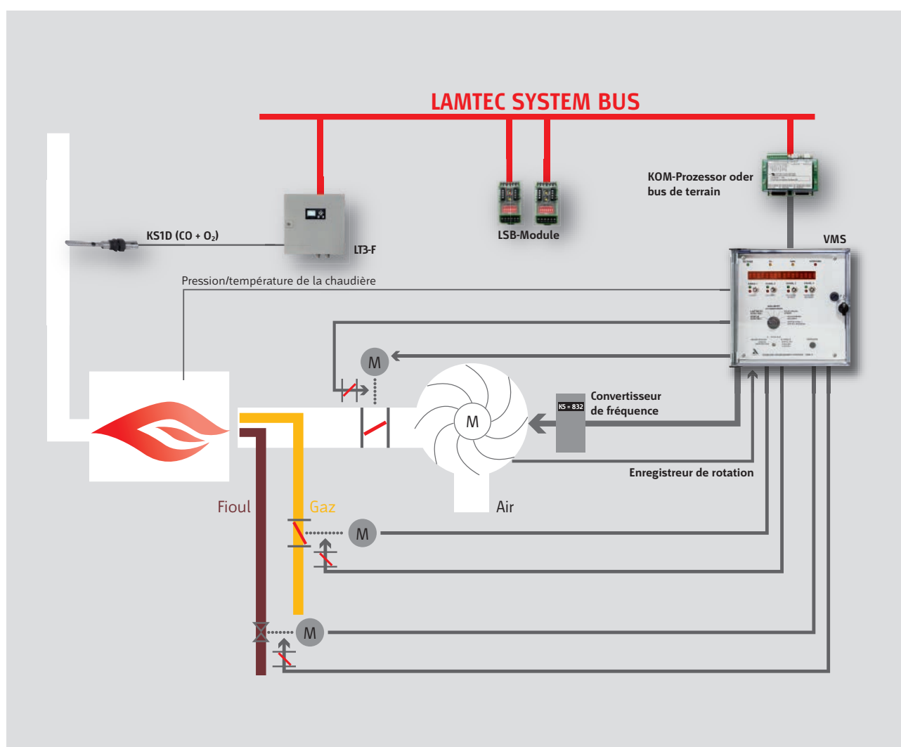
Aperçu fonctionnel VMS.
